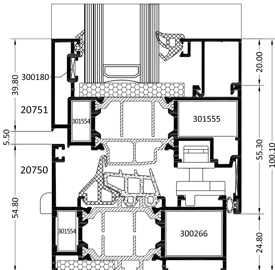
SECCIÓN S1
